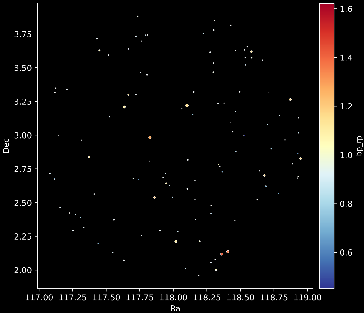
GALAH DR4 Field: [6686] Stars: 112
