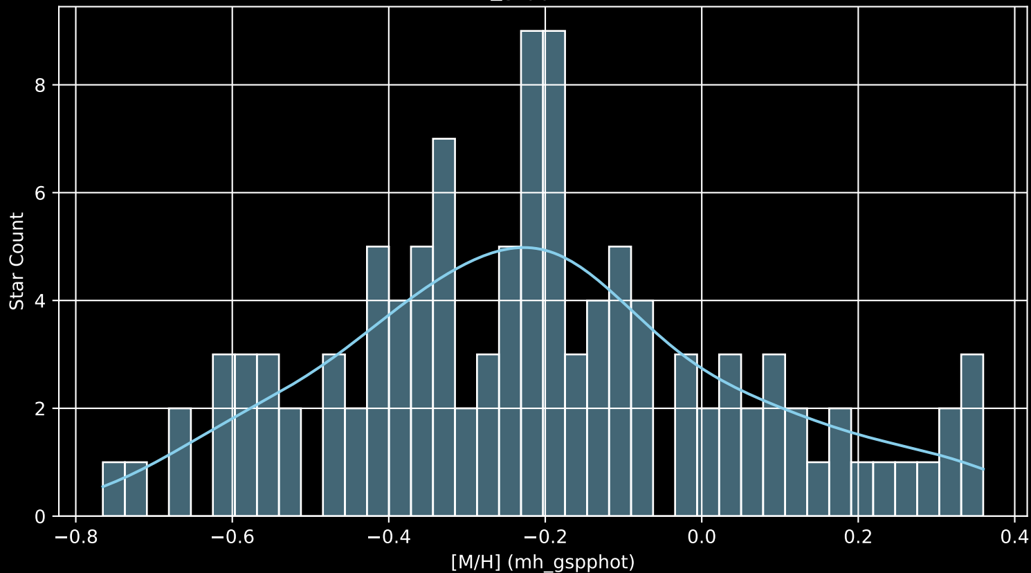
GALAH DR4 Field: [6686] [M/H] (mh_gspphot) (n= 112)
