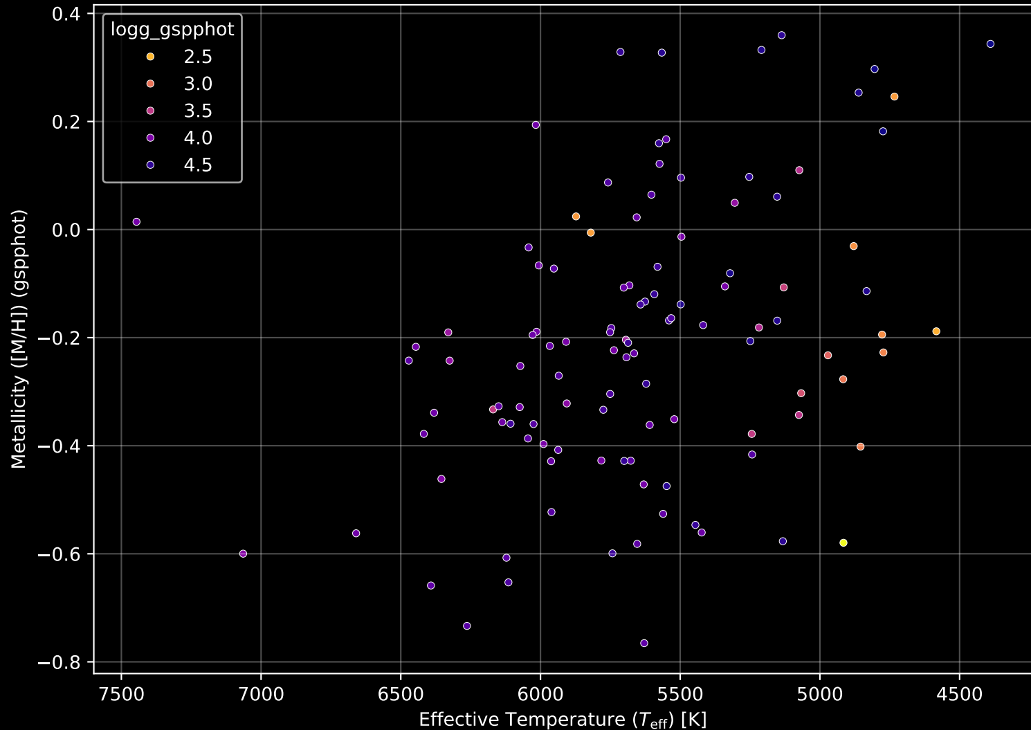
GALAH DR4 Field: [6686] Stellar Population Parameters (n= 112)
