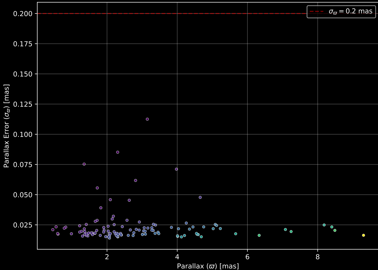
GALAH DR4 Field: [6686] Parallax Quality (n= 112)
